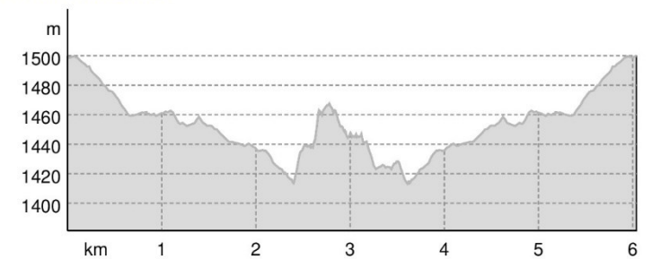
Profilo altimetrico
